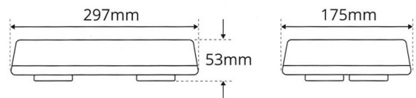
MPL300 Abmessungen in mm.
